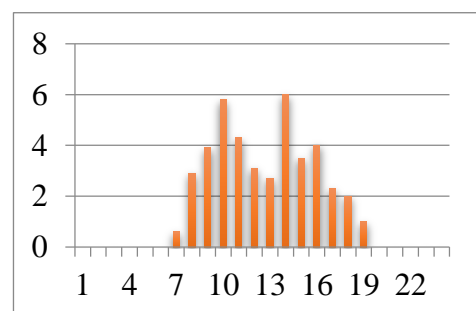
شکل (۱۱): نمودار تغییرات قدرت خروجی سلول خورشیدی با ۲۵٪ کاهش در تابش خورشید نسبت به حالت نامی به‌دست‌آمده با Homer
