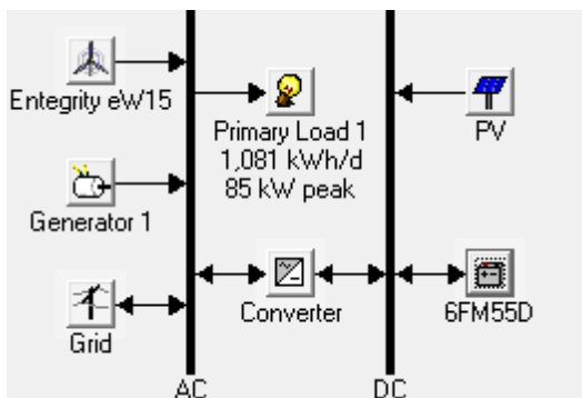
شکل (۱): مدل ریزشبه مدنظر در نرم‌افزار Homer
