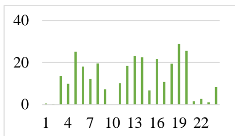
شکل (۵): قدرت خروجی توربین بادی بر حسب کیلووات طی
