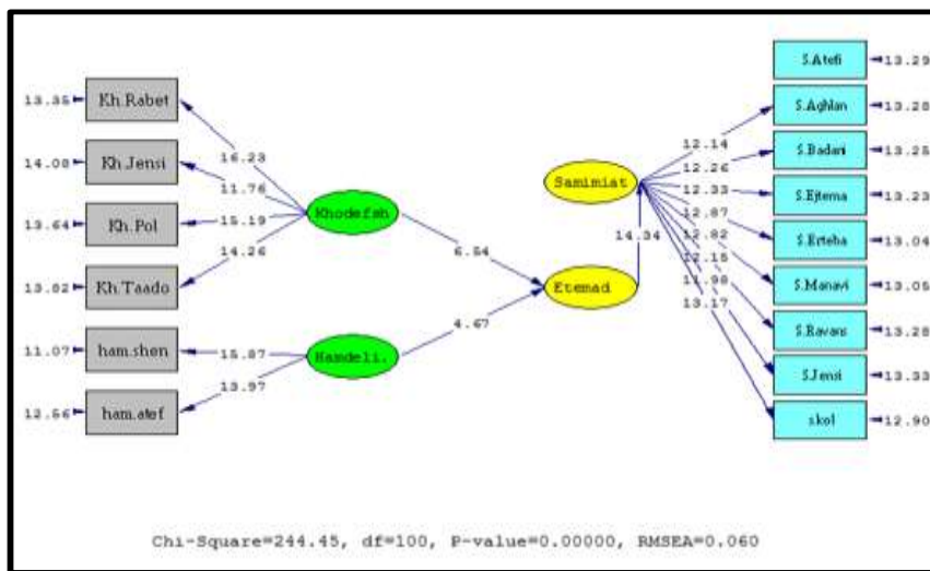
شکل ۱: نمودار مدل معادلات ساختاری آزمون شده در حالت معناداری
