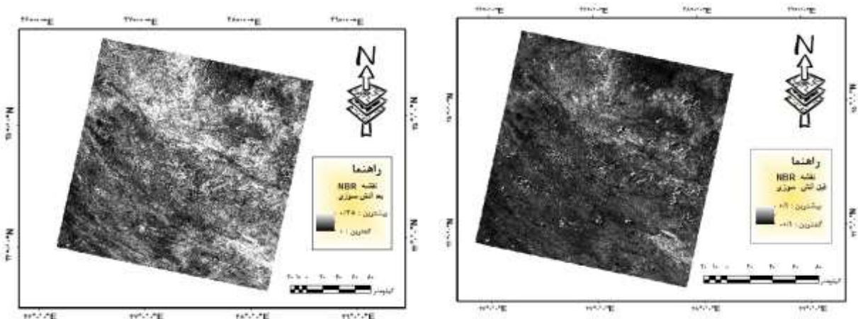
شکل (۴) نقشه شاخص NBR قبل از آتش‌سوزی (سمت راست) و بعد از آتش‌سوزی (سمت چپ)
