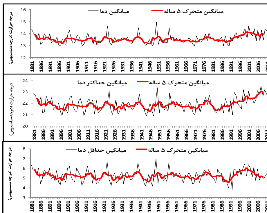
شکل ۷) نمایش میانگین، میانگین حداکثر و میانگین حداقل دمای سالانه بازسازی شده طی ۱۳۱ سال گذشته همراه با میانگین متحرک ۵ ساله آنها، در منطقه دنا (۱۸۸۱-۲۰۱۱)
