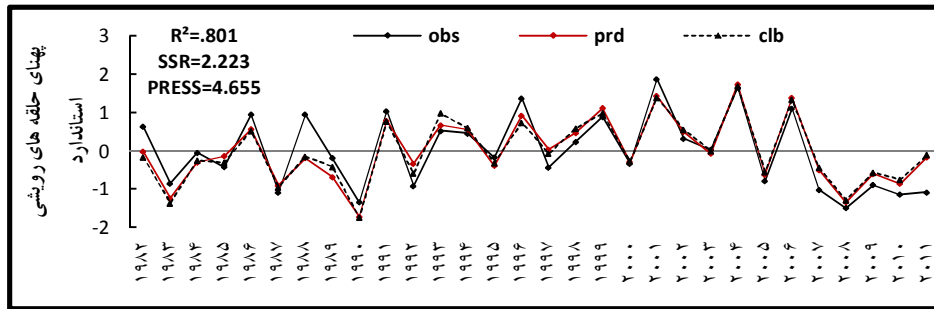
شکل ۶) برهم گذاری منحنی مقادیر واقعی (obs)، برآورد (prd) و کالیبراسیون (clb) برای گونه بلوط ایرانی منطقه دنا در طول ۳۰ سال اخیر (۱۹۸۲-۲۰۱۱)
