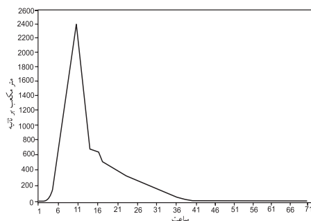
شکل ۷: هیدرو گراف سیل ایستگاه سرمقسم
