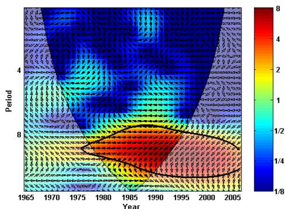
شکل ۶: تبدیل موجک متقاطع بین نوسان‌های بارش‌های سالانه دریاچه ارومیه و لکه‌های خورشیدی
