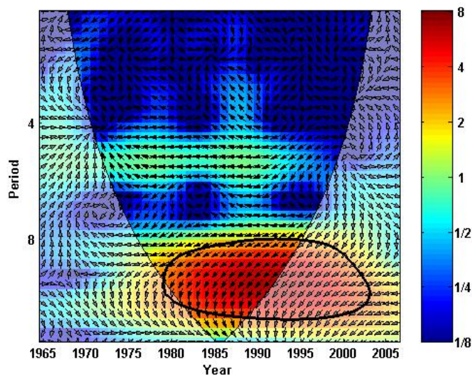
شکل ۱۰: تبدیل موجک متقاطع بین حجم سالانه رواناب‌های ورودی به دریاچه ارومیه و لکه‌های خورشیدی
