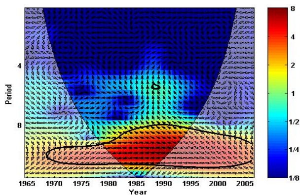
شکل ۴: تبدیل موجک متقاطع بین نوسانهای سطح آب دریاچه ارومیه و لکه‌های خورشیدی
