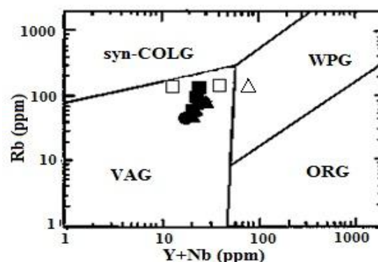
شکل ۱۵- موقعیت نمونه‌های گرانیتوئید ملاطالب بر روی نمودار تفکیک‌کننده محیط‌های تکتونیکی (Pearce et al. , 1984) (نشانه‌ها مشابه شکل ۱۰ است).
