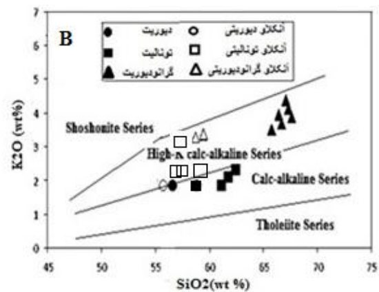
شکل ۴-۱ (A) موقعیت سنگ‌شناختی نمونه‌های گرانیتوئیدی ملاطالب در نمودار R2-R1 (De La Roche et al. , 1980)؛ (B) پراکنندگی نمونه‌های بررسی شده در سری‌های کالک‌آلکان و کالک‌آلکان پتاسیک بالا در نمودار K_2O در برابر SiO_2 (Rickwood, 1989).
