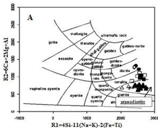
شکل ۴-۱ (A) موقعیت سنگ‌شناختی نمونه‌های گرانیتوئیدی ملاطالب در نمودار R2-R1 (De La Roche et al. , 1980)؛ (B) پراکنندگی نمونه‌های بررسی شده در سری‌های کالک‌آلکان و کالک‌آلکان پتاسیک بالا در نمودار K_2O در برابر SiO_2 (Rickwood, 1989).
