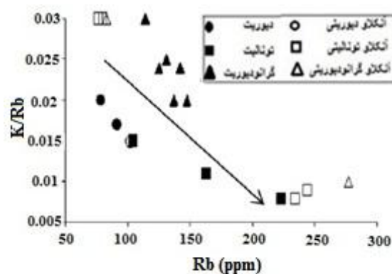
شکل ۱۰- روند کاهش‌ی نمونه‌های منطقه در نمودار K/Rb در برابر Rb که بیانگر تأثیر پدیده تفریق کریستالی در تشکیل توده گرانیتوئید ملاطالب است.
