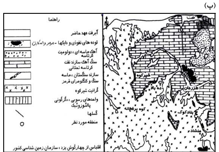
شکل ۱- الف) جایگاه اسکارن‌های مورد مطالعه در نوار ماگماتیسیم سنوزوییک ایران مرکزی (F= فشارک و S= شیرکوه)، ب) نقشه زمین‌شناسی اسکارن فشارک اصفهان (برگرفته از نوربهبشت، ۱۳۷۰)، پ) نقشه زمین‌شناسی اسکارن شیرکوه یزد (برگرفته از مکی زاده، ۱۳۸۷ با تغییرات) (مقیاس ۱:۲۵۰۰۰۰)
