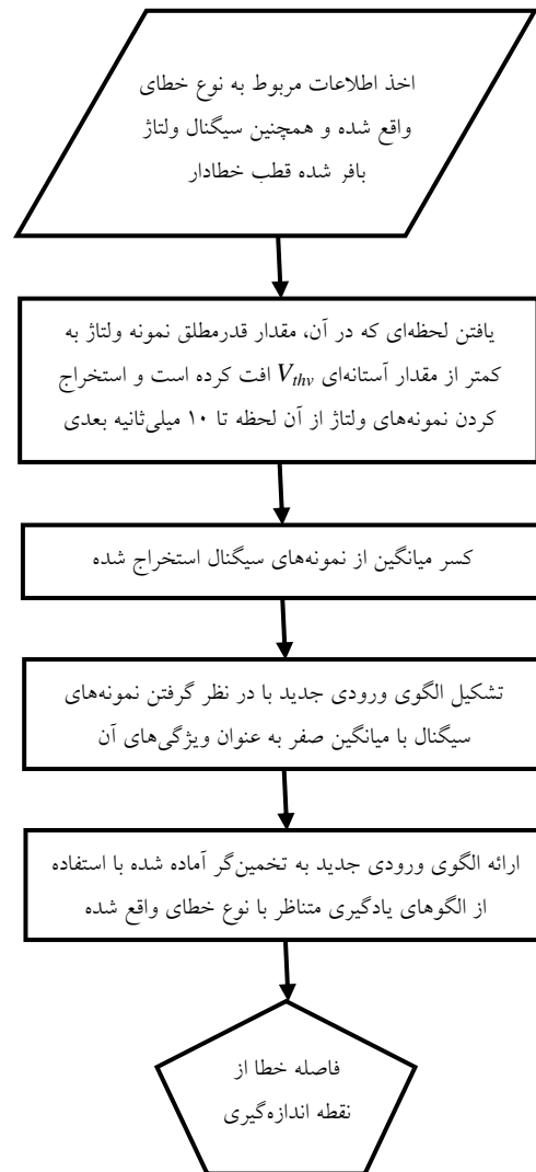
شکل (۳): الگوریتم کلی روش پیشنهادی برای مکان‌یابی خطا
