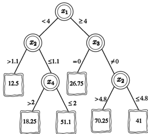
شکل (۲): یک نمونه از درخت تصمیم رگرسیونی
